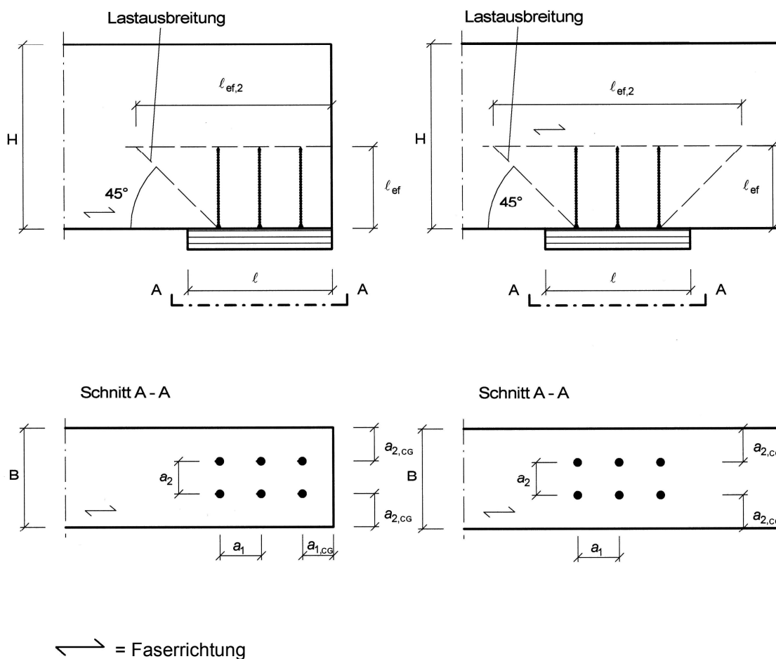
Abbildung A.3.1: Verstärktes Endauflager (links) und verstärktes Zwischenaullager (rechts)
