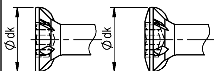
Kleiner (Linsensenk-) Kopf
