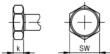
Sechskantkopf
