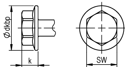
Sechskantkopf mit Bund
