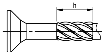
Schafffräser
