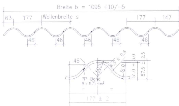
Bild 1 c: Wellplatten P6 mit PP-Bändern: Querschnittsabmessungen und Lage Bänder
