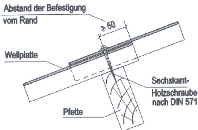
Bild 3b: Befestigung auf einer Holzpforte mit einer Sechskant-Holzschraube nach DIN 571
